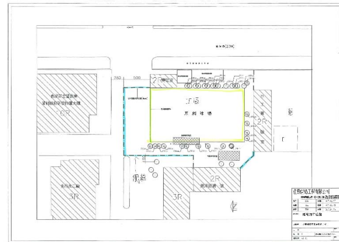
【立體機車停車場圍籬搭設範圍】
