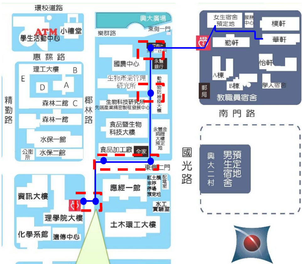
【網路光纖及電話纜線線路佈線示意圖】
