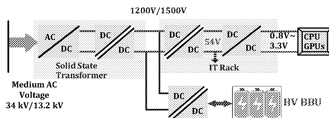
圖 1 未來 AI 伺服器系統之供電架構
